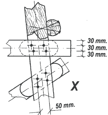
Knotenpunkt genagelt mit 4 Nägeln 4,2/120 je Anschluss
